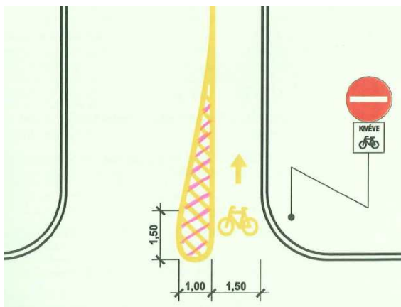
7. ábra: Kerékpáros bejárat kapu burkolati jellel
