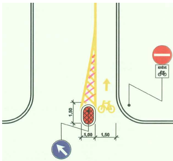
8. ábra: Kerékpáros bejárat kapu épített szigettel
