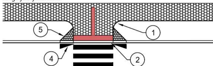
118. ábra: Járda csatlakozása gyalogos-átkelőhelyhez zóldsáv esetén (példa)
