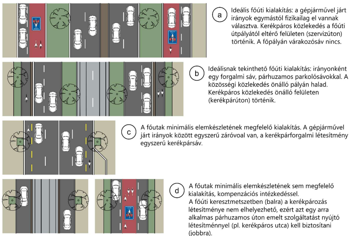
18. ábra A főúti elemkészlet bemutatása
