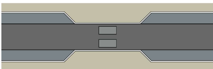
71. ábra: Busszal „megközölhető” kialakítású küszöb.
