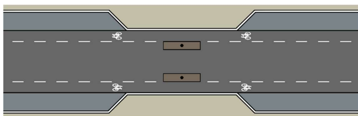
78. ábra: Egy nyomra szűkített útpálya nyitott kerékpársáv esetén a nyitott kerékpársáv megszakítása nélkül (példa)
