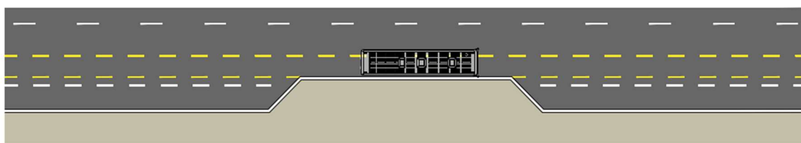
142. ábra: Félszigetes megállóhely kerékpársávval (példa)
