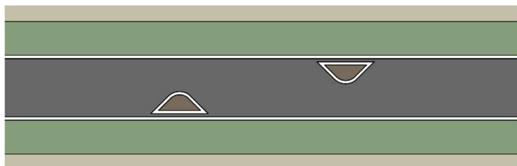
77. ábra: A járóvonal elhúzása „úszó” szigetekkel (vagy ideiglenesen egyéb forgalomtechnikai elemekkel, virágládával), a burkolt keresztmetszet oldalirányú szűkítésével, elsősorban kertvárosi környezetben (példa)
