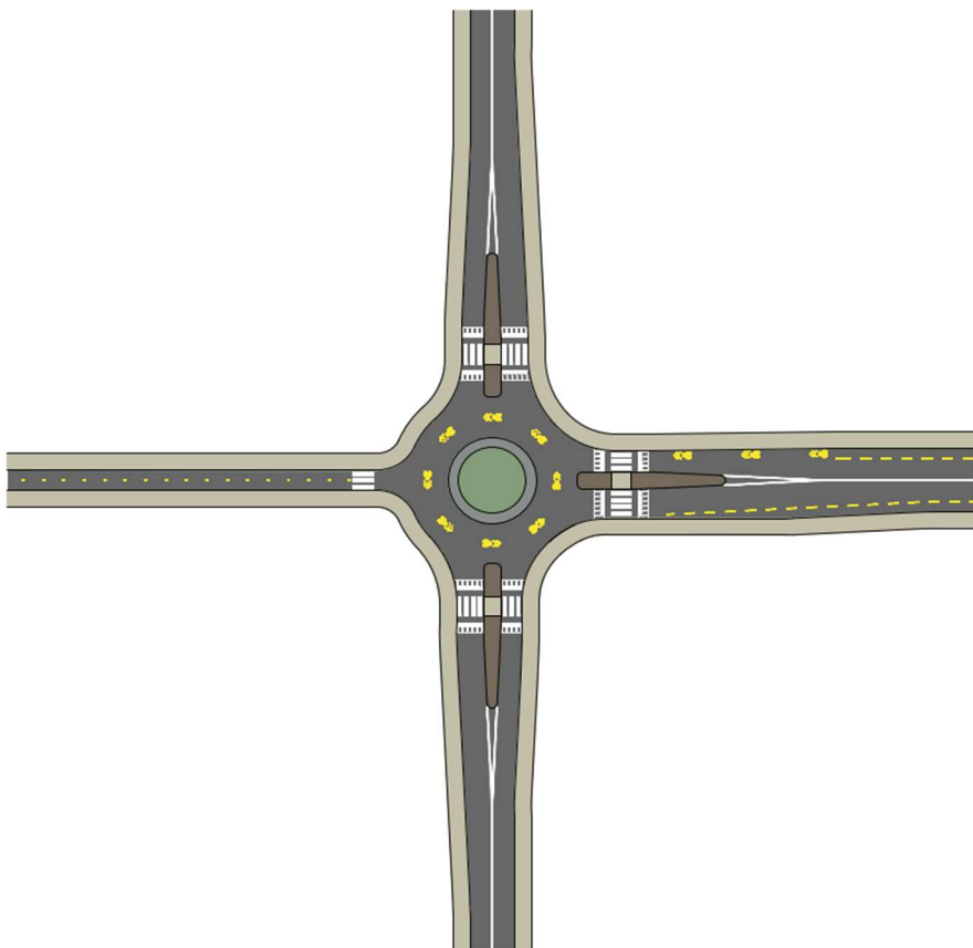
94. ábra: Kisméretű körforgalom városias környezetben, helyi utak és gyűjtőutak csomópontjában (példa)
