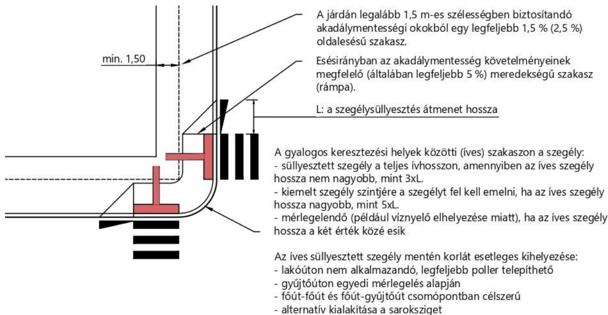
115. ábra: Szegélyszüllyesztés kialakítása széles járdán oldalirányú rámpával (példa)
