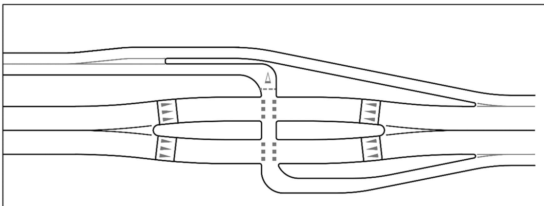
53. ábra: Átmenet kétirányú kerékpárút és kerékpársávok között középszigettel és pályaszint emeléssel (példa)
