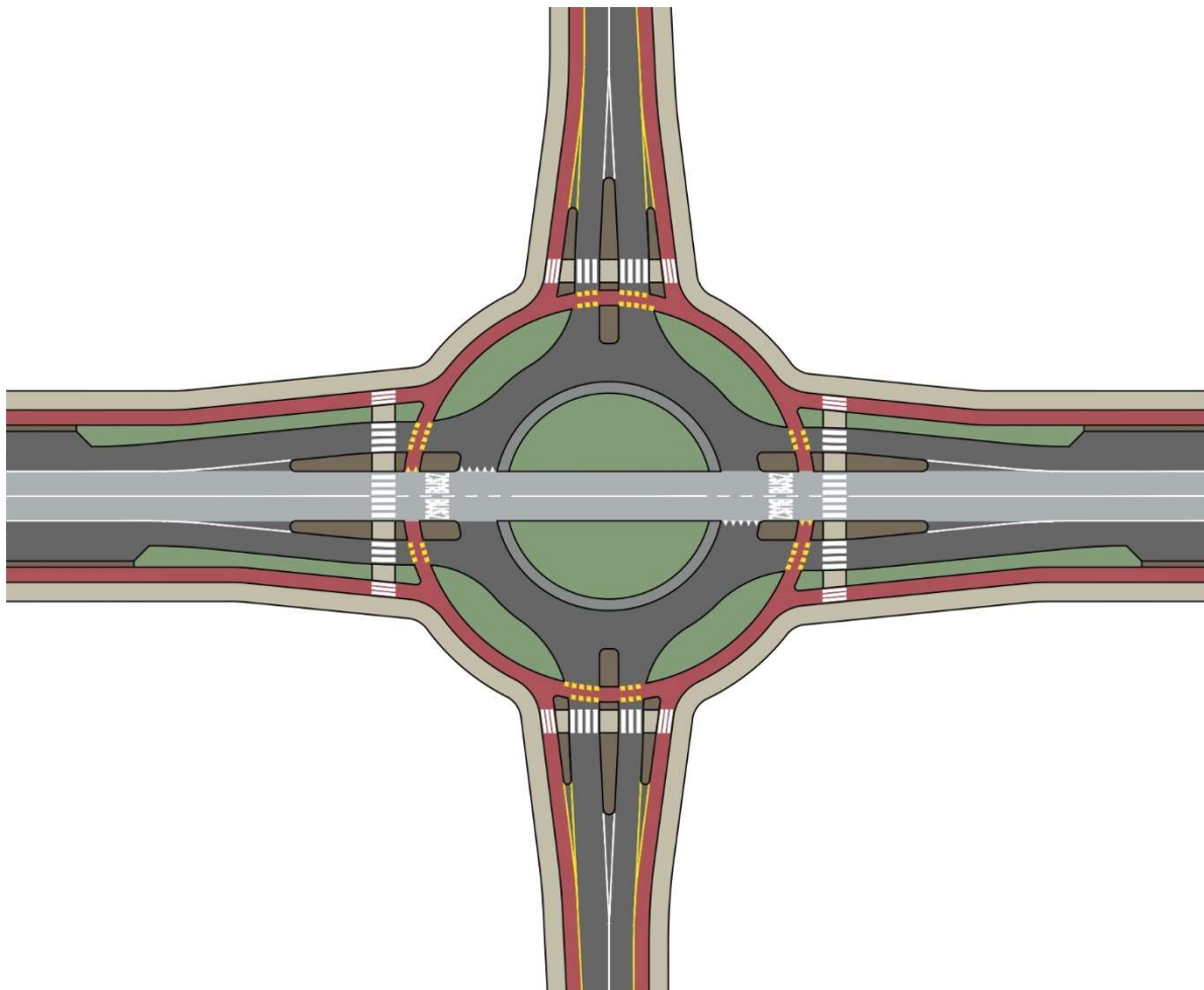
130. ábra: Közösségi közlekedési pálya átvezetése körforgalmon keresztül (példa)
