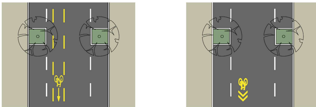
34. ábra: Kerékpárral kétirányú utca ellenirányú kerékpársávval (balra) és kerékpársáv nélkül (jobbra) (példák)
