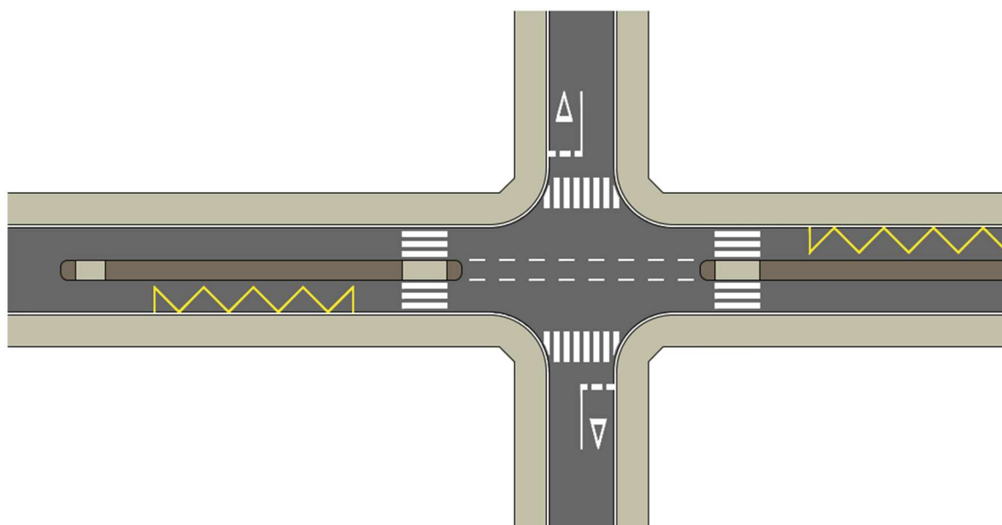
146. ábra: Folytonos szigettel védett megálló csomópontban (példa)
