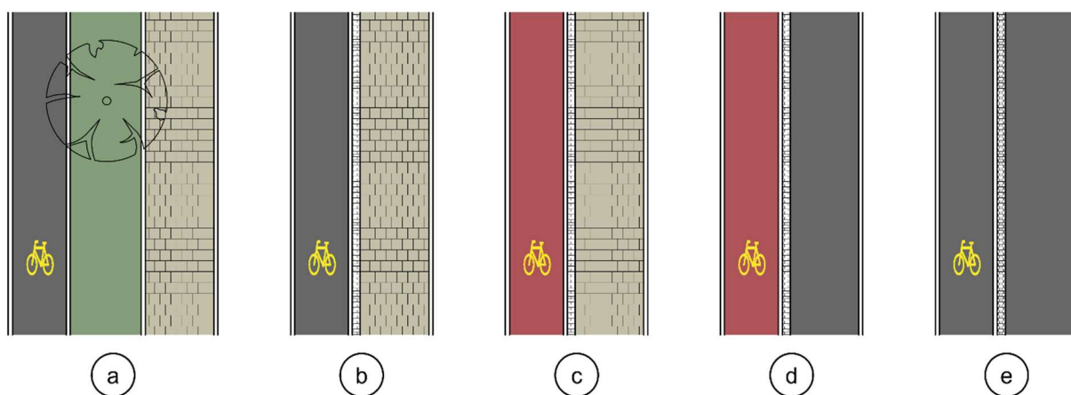
26. ábra: A kerékpáros és gyalogos forgalom elválasztását hangsúlyozó különböző lehetőségek
