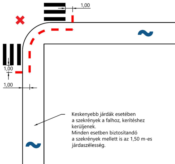
160. ábra: Egyszerű járdasarok berendezési sáv, zöldsáv, kerékpárút nélkül
