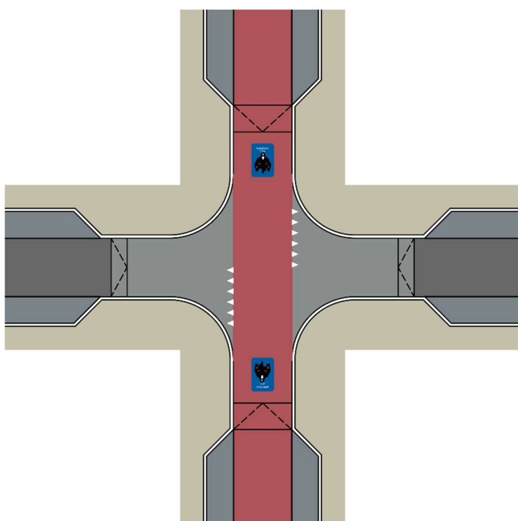
86. ábra: Kerékpáros utcának kijelölt út csomópontja lakóúti környezetben (példa)
