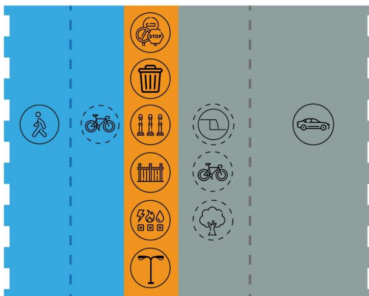
8. ábra: Térségi jelentőségű út keresztmetszete
