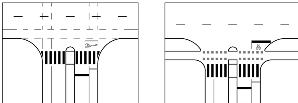
50. ábra: Közvetett kerékpáros kapcsolat kialakítása kerékpársáv (balra) és kerékpárút esetén (jobbra). Közvetett kerékpárút esetén a kerékpársávhoz hasonlóan lehet eljárni.
