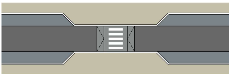
106. ábra: Gyalogos-átkelőhely lakóúti környezetben, pályaszint-emelésen
