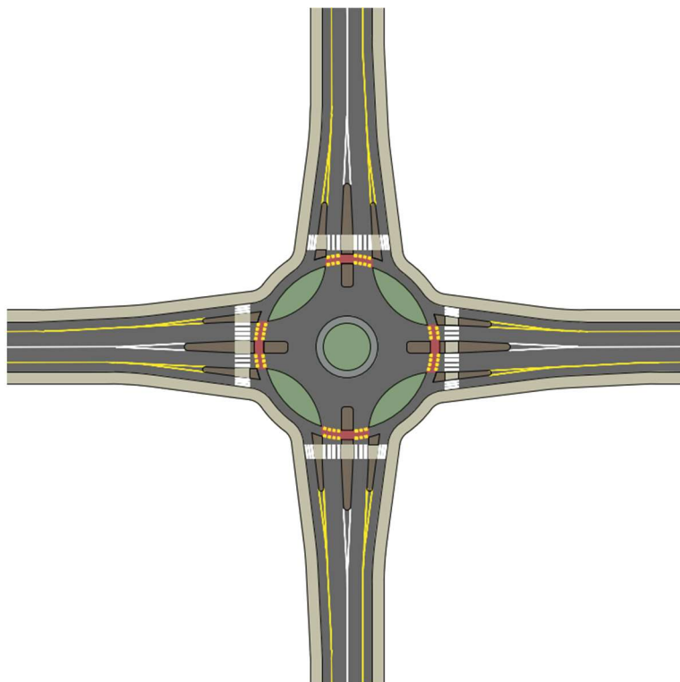
95. ábra: Városias környezetben alkalmazandó körforgalom fő- és gyűjtőúti környezetben (példa)
