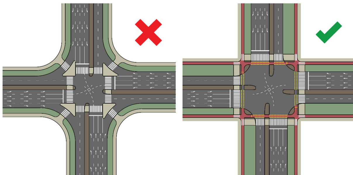
105. ábra: Hiánytalanul (középszigetekkel) kialakított főút-főút csomópont háromszögszigetekkel (balra). Magyarországon a hiányos, sziget nélküli elrendezés terjedt el. Kerülendő elrendezés. Kompakt főúti csomópont (jobbra).
