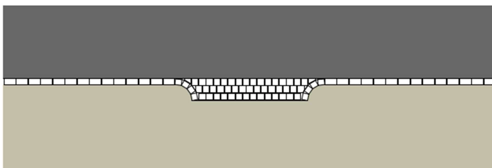
152. ábra: Igényes megoldások kapubeállók esetében (fent: gránit kapubeálló szegély, közepén: 3 sor ferde síkban és néhány sor vízszintes síkban fektetett nagykockakő rámpával, alul: 3 sor ferde síkban fektetett nagykockakő rámpával)
