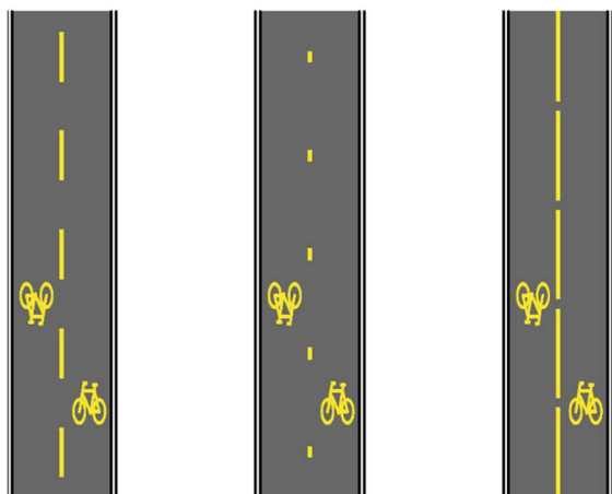
65. ábra: Kerékpárút burkolati jelei: a megszokott terelővonalal (balra), ritkított terelővonalal (középen) és sűrített terelővonalal (jobbra)
