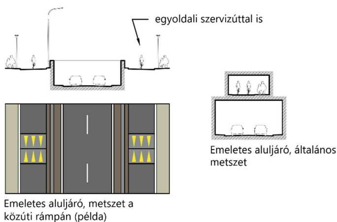
64. ábra: Kétszintes alujáró kialakítása keresztmetszeti kötöttségek esetén (példa)
