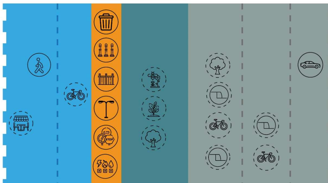
9. ábra: Városi főút keresztmetszete
