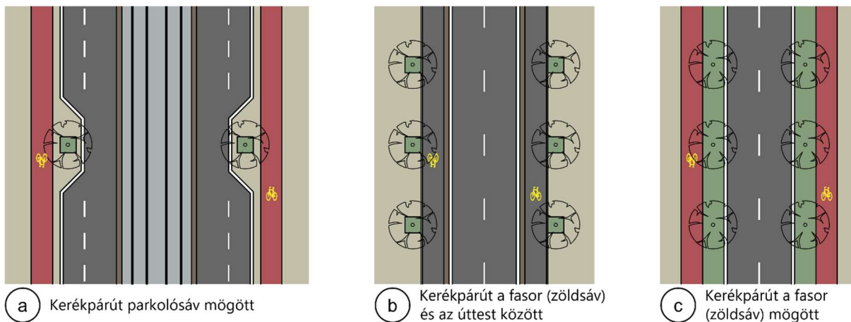
25. ábra: Elválasztott gyalog- és (egyirányú) kerékpárút kialakítása (példa)
