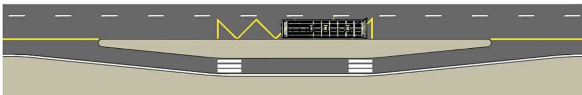
144. ábra: Peronszigetes megállóhely kerékpársávval (példa)
