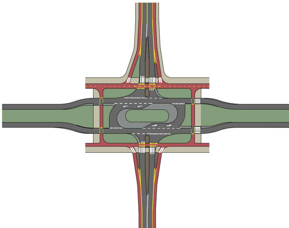
98. ábra: Voorrangsplein csomópont, szabványosított kialakítás
