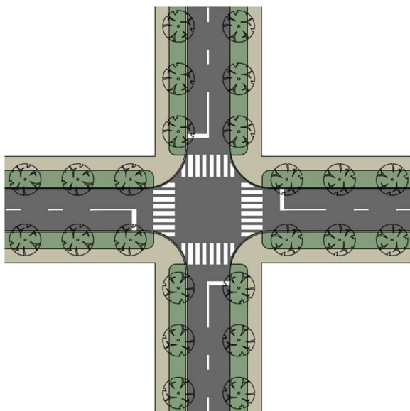
102. ábra: Jelzőlámpás csomópont szűk keresztmetszetű környezetben, a csomóponthoz közel húzott gyalogos-átkelőhellyel (példa)
