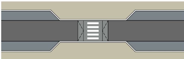
73. ábra: Gyalogos-átkelőhely emelt pályaszinten (példa)
