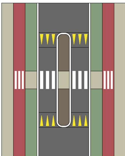
107. ábra: Gyalogos-átkelőhely ideális kialakítása (példa)
