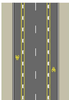
29. ábra: Védett kerékpársáv forgalomtechnikai elemekkel elválasztva (példa)
