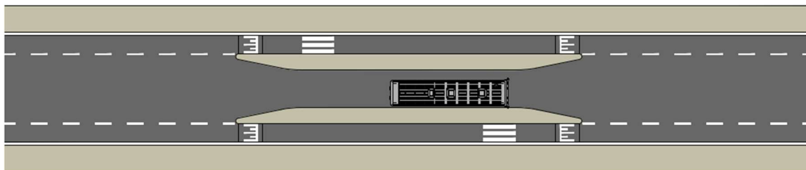
151. ábra: Példa egy nyom szélességre szűkített útpályán kialakított megállóhely kialakítására
