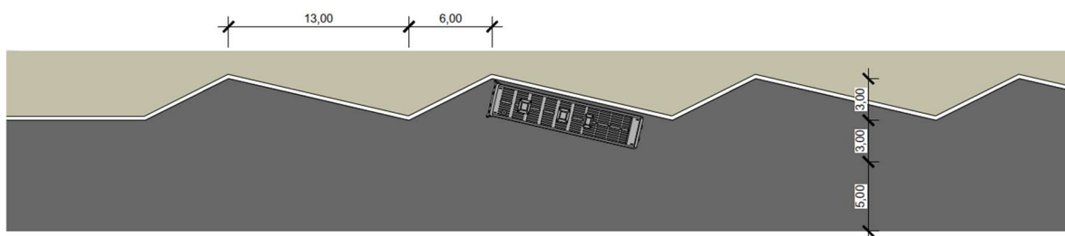
149. ábra: Fűrészfogas kocsiállások szóló buszok figyelembevételével
