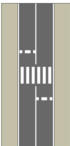
111. ábra: Kerülendő az az elrendezés, ahol a gyalogos-átkelőhelyet a forgalomtechnikai jelzéseken kívül semmi nem védi
