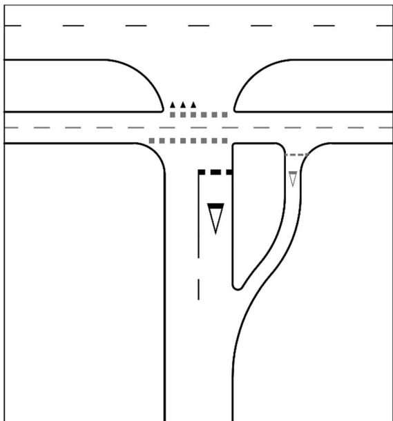
48. ábra: Kétirányú kerékpárúttal való kapcsolat segítése kerékpárúti felhajtóval
