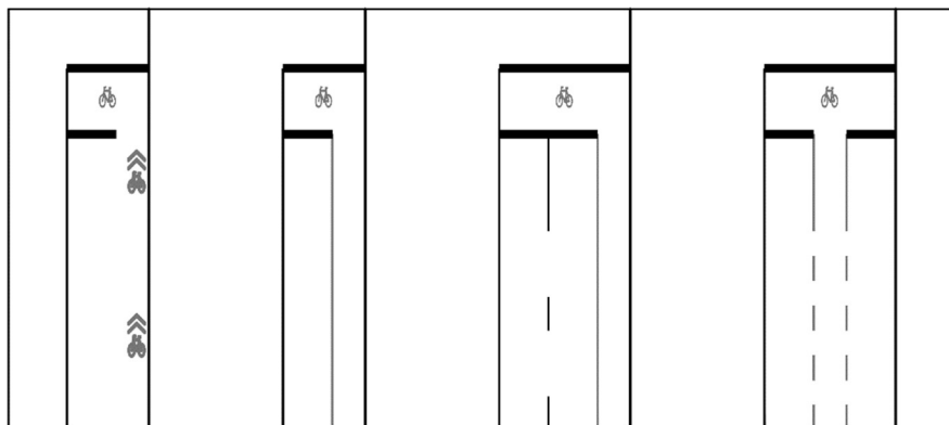
51. ábra: Előretolt kerékpáros felállóhely kialakítási lehetőségei (példa)
