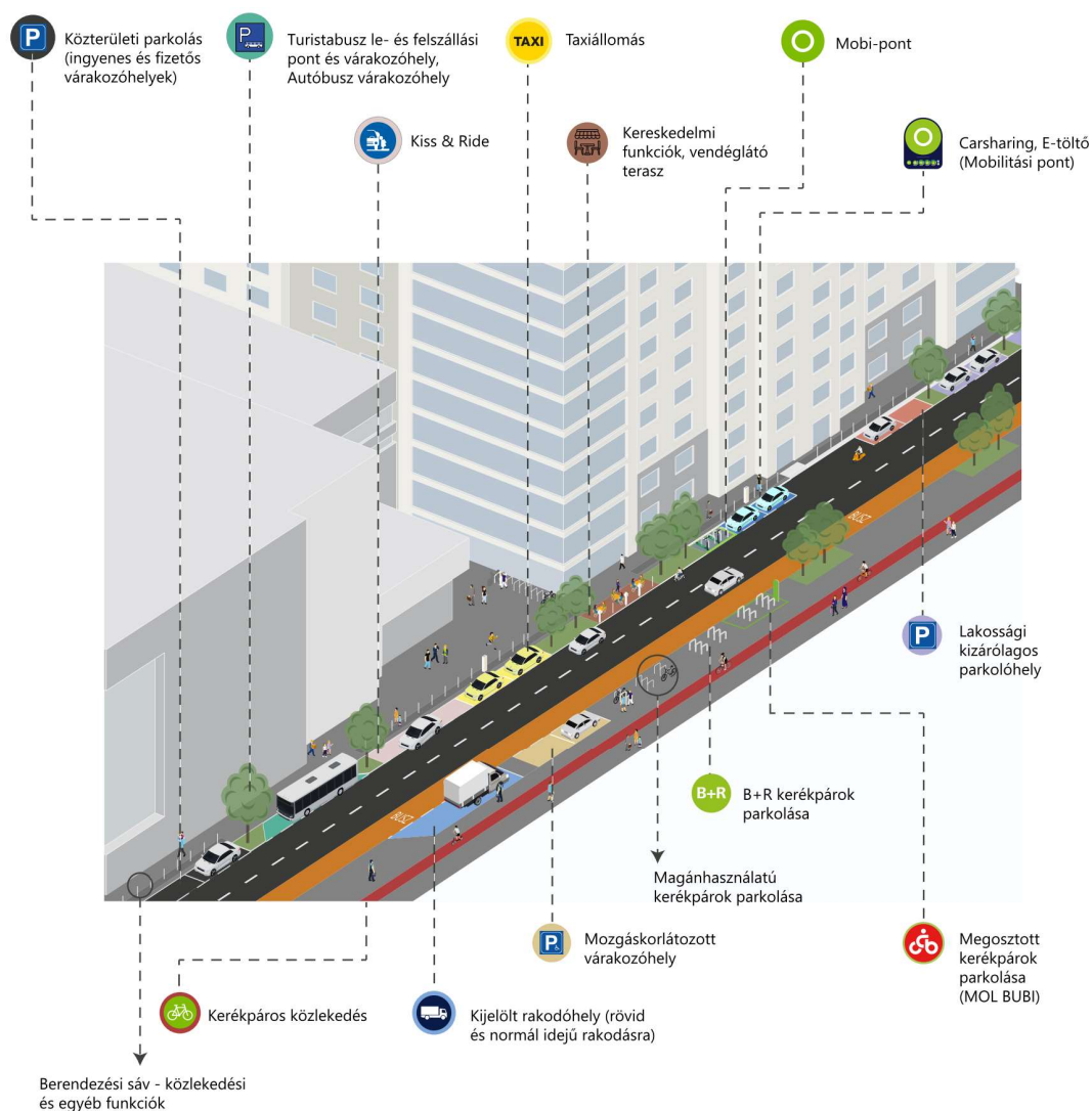
17. ábra: Szegélyzóna magyarázó ábra
