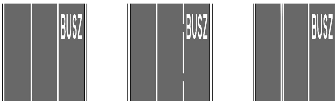
131. ábra: Buszsáv jelölésének helytelen (balra) és helyes módjai (középen, jobbra)
