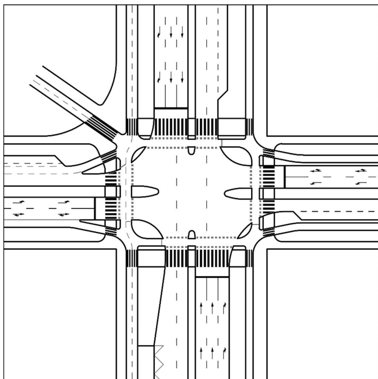
46. ábra: Többféle kerékpárforgalmi létesítmény közötti egyszerű kapcsolatot biztosító csomópont kerékpárút átvezetéssel. A csomópontban kapcsolódik kétoldali egyirányú kerékpárút, kétirányú kerékpárút, kerékpársáv és ötödik ágként egy további kerékpárút is. (példa)
