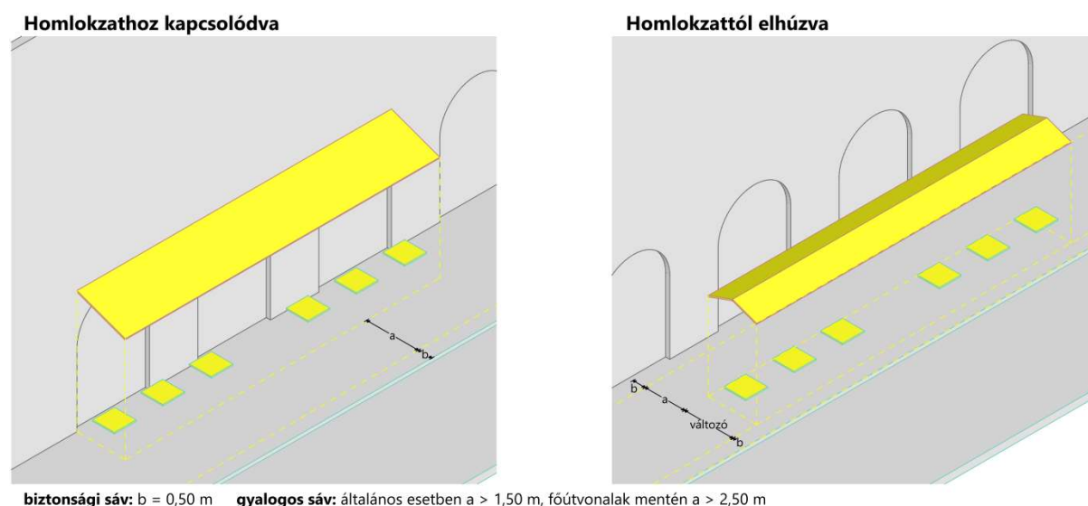
6. ábra: Teraszok elhelyezési lehetőségei
