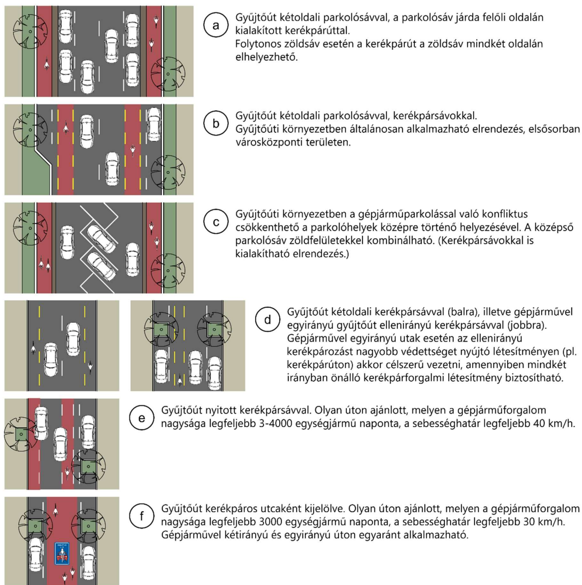
23. ábra: A kerékpáros közlekedés helye gyűjtőúti környezetben (példák)
