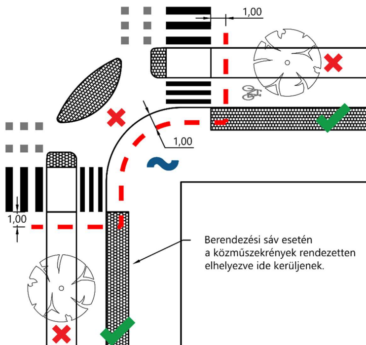
158. ábra: Sarok zöldsávval, kerékpárúttal, járdával
