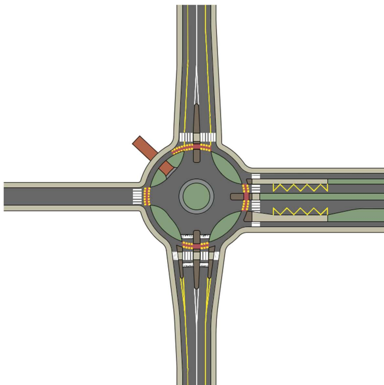
96. ábra: Példa különböző módon csatlakozó ágakra, ingatlan csatlakozásra és buszmegálló kialakítására körforgalomban
