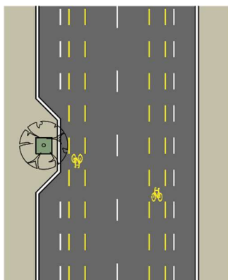
30. ábra: Kerékpársáv kialakítása (példa)
