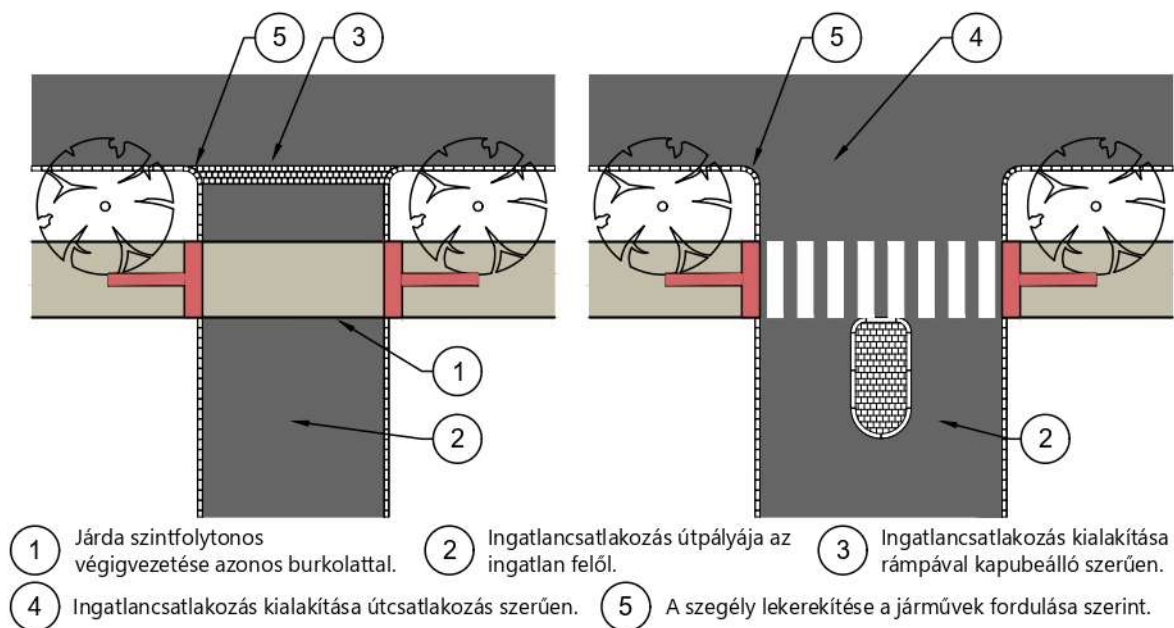
126. ábra: Nagyforgalmú kapubeállók kialakítási lehetőségei (minta)
