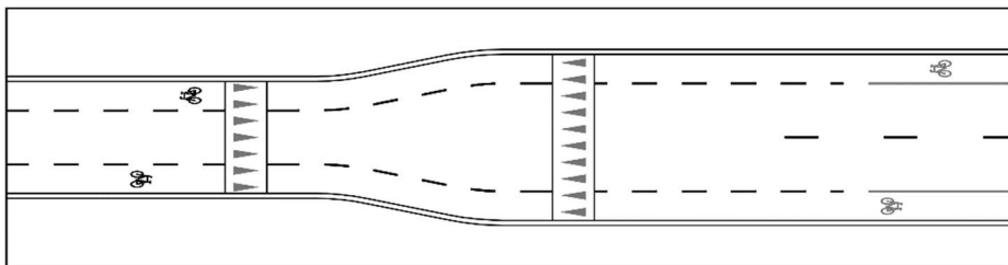
55. ábra: Nyitott kerékpársáv kezdete pályaszint-emelésen (példa)
