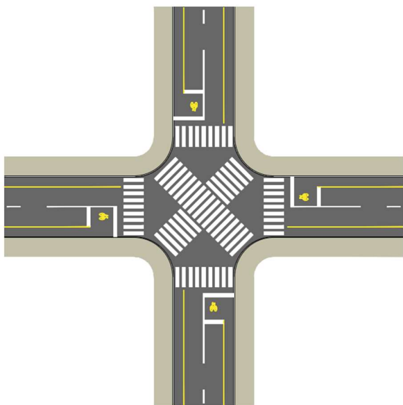
104. ábra: Jelzőlámpás csomópont szűk keresztmetszetű környezetben, átlós irányú gyalogos-átkelőhelyekkel (példa)
