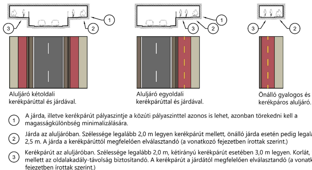
63. ábra: Alujárók kialakítási lehetőségei (példák)
