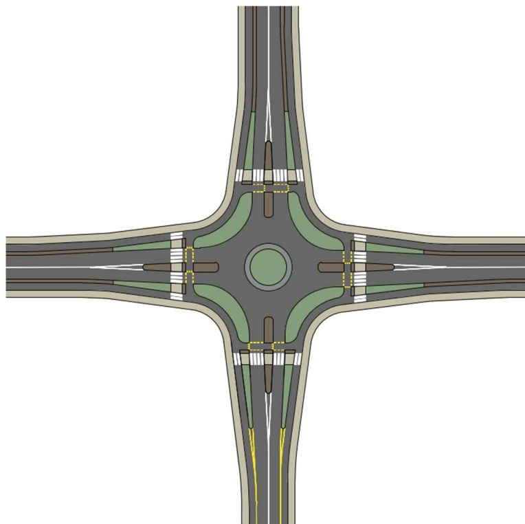
97. ábra: Külső zónában és külterületen alkalmazandó körforgalom elvi sémája a kerékpárutak rátörésével, alárendelésével (példa)
