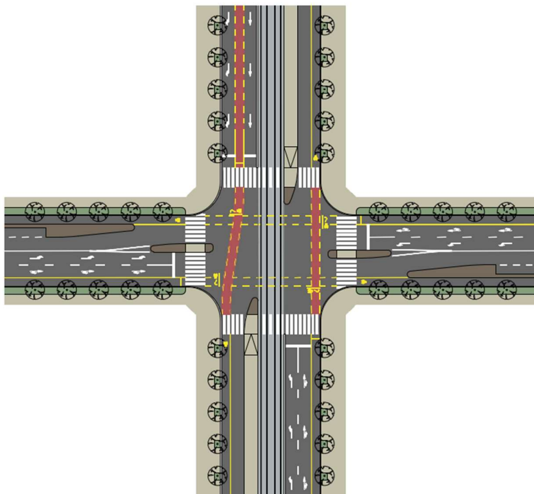
99. ábra: Fő- és gyűjtőúti környezetben kialakított jelzőlámpás csomópont kialakítása, a csomópontban közösségi közlekedési pályával, kerékpársávok átvezetésével, elsősorban városközponti területen (példa)
