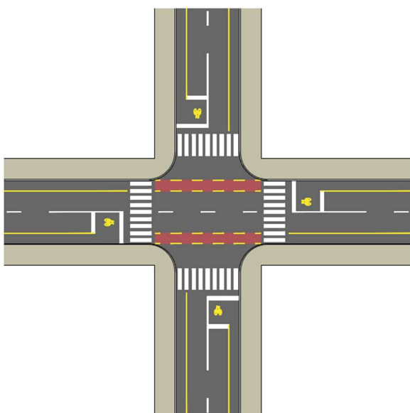
103. ábra: Jelzőlámpás csomópont szűk keresztmetszetű környezetben, kerékpársávokkal (példa)
