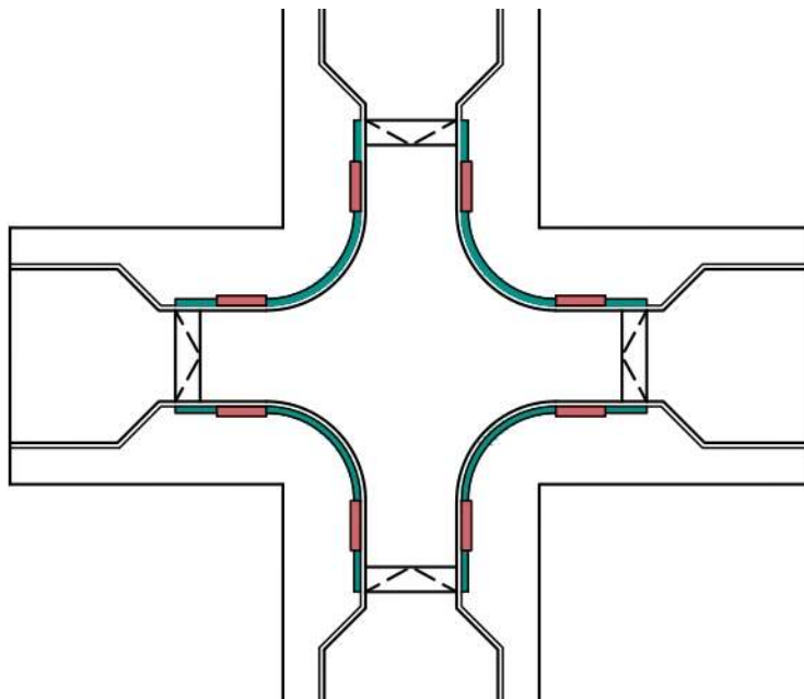
117. ábra: Kiemelt csomópontban a vakok és gyengénlátók számára megfelelő kialakítás a gyalogos keresztezésre nem ajánlott helyeken kontrasztos és tapintható burkolattal (az ábrán zöld színnel) (példa)
