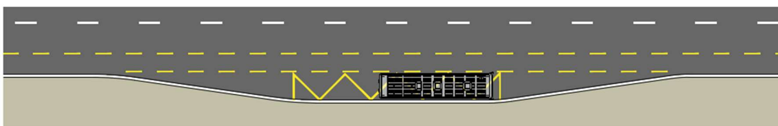
137. ábra: Öbölben kialakított megállóhely gyűjtőúton, kerékpársávval (példa)
