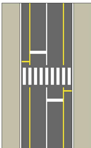
110. ábra: Gyalogos-átkelőhely megfelelő szintű kialakítása jelzőlámpás szabályozással
