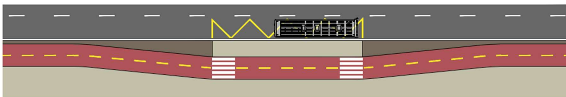
145. ábra: Peronszigetes megállóhely kétirányú kerékpárúttal (példa)
