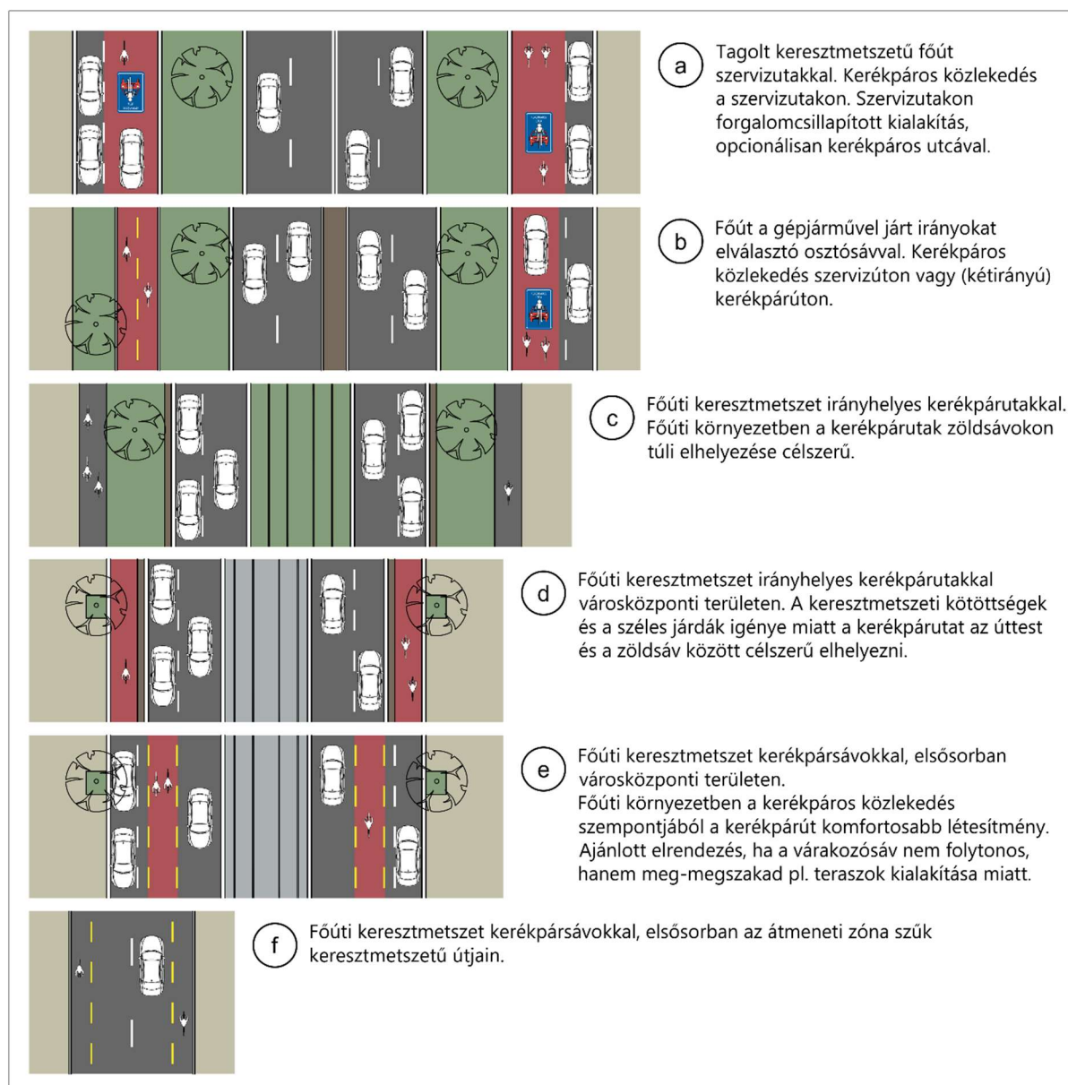
24. ábra: A kerékpáros közlekedés helye főúti környezetben (példák)
