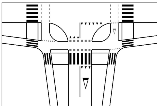
67. ábra: Példa cápa fog burkolati jel alkalmazására
