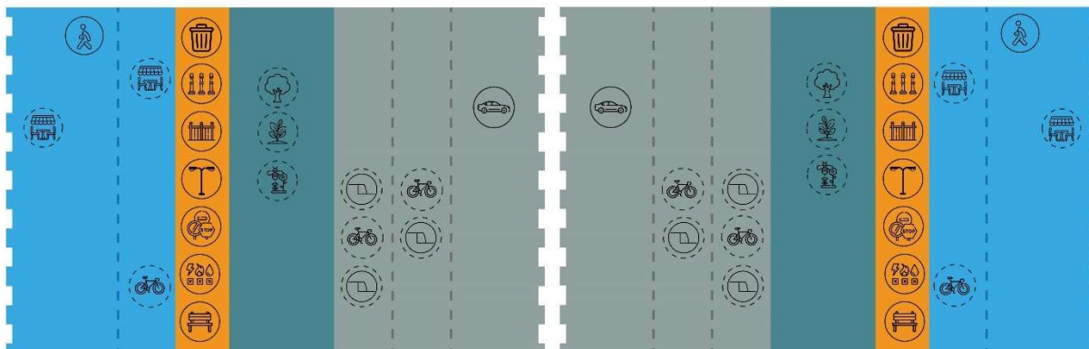
14. ábra: Kerületközponti utca keresztmetszete
