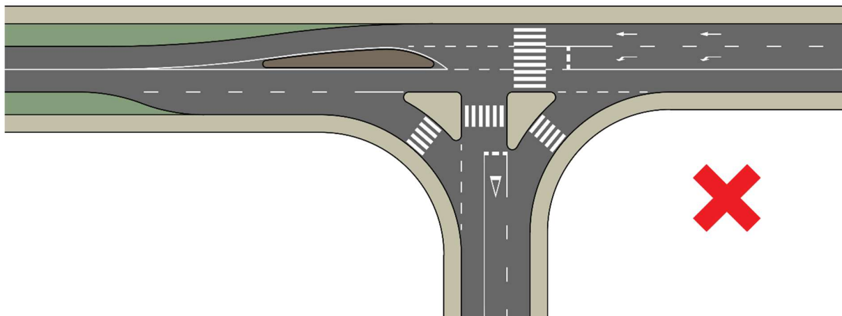
92. ábra: Tiltott elrendezés. Főirányban osztályozós torkolat található, a mellékirány pedig szerkesztési hibával terhelt (példa).
