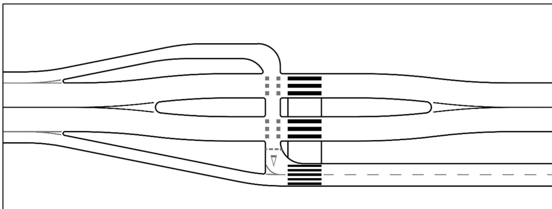
52. ábra: Átmenet kétirányú kerékpárút és kerékpársávok között középszigettel (példa)
