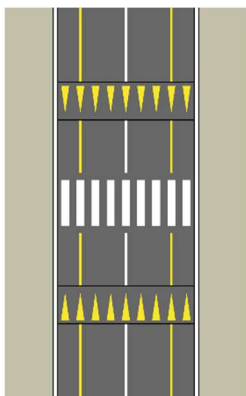
68. ábra: Az UME szerinti burkolati jel helyes alkalmazása aszfalt burkolatú rámpák esetében (példa)
