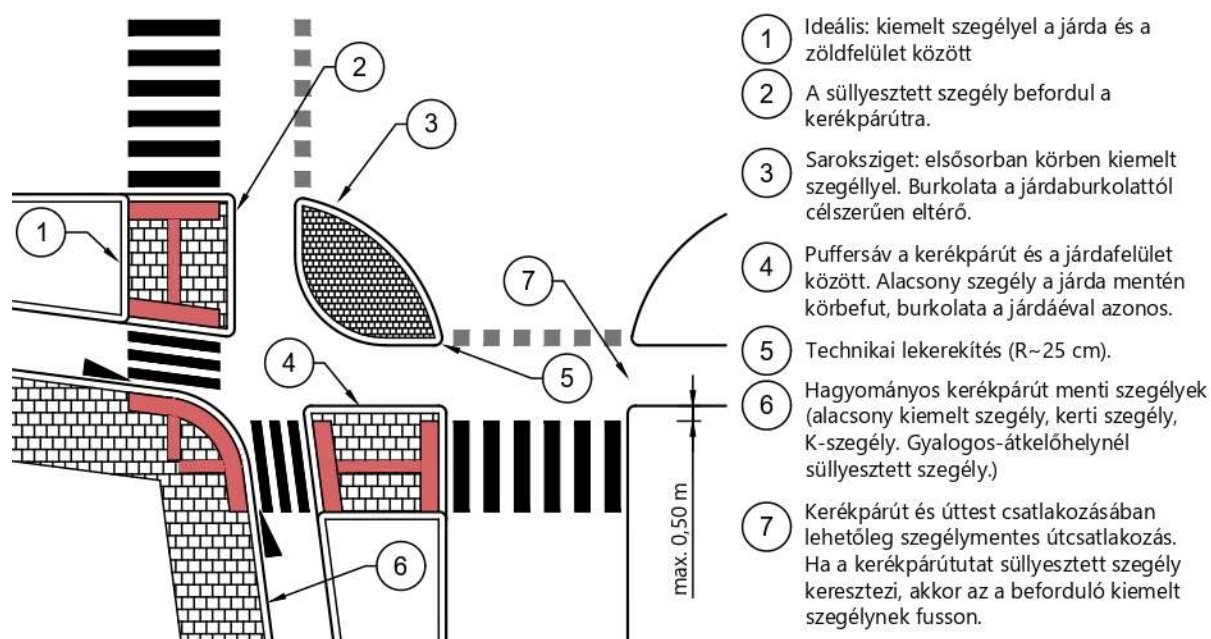
120. ábra: Utcasarok kialakítása kerékpárút esetén a gyalogos és kerékpáros felületek között puffersáv nélkül (minta)
