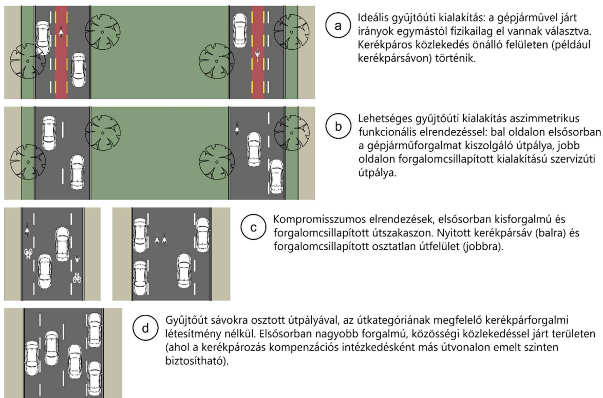
19. ábra: A gyűjtőúti elemkészlet bemutatása
