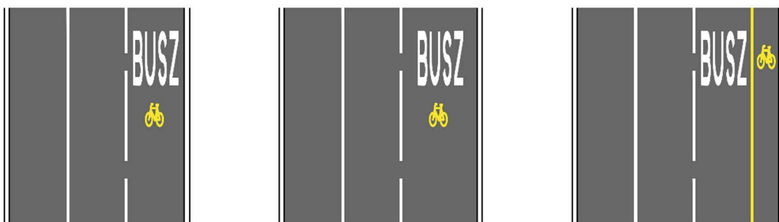
127. ábra: Közös busz- és kerékpársáv maximum 3,25 m szélességgel (balra), közös busz- és kerékpársáv legalább 4,25 m szélességgel (középen), önálló busz- és önálló kerékpársáv (jobbra)
