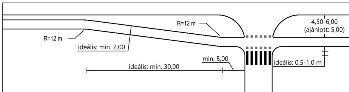
42. ábra: Kerékpárút 5 m-re elhúzott átvezetéssel egyszerű torkolatban (példa)
