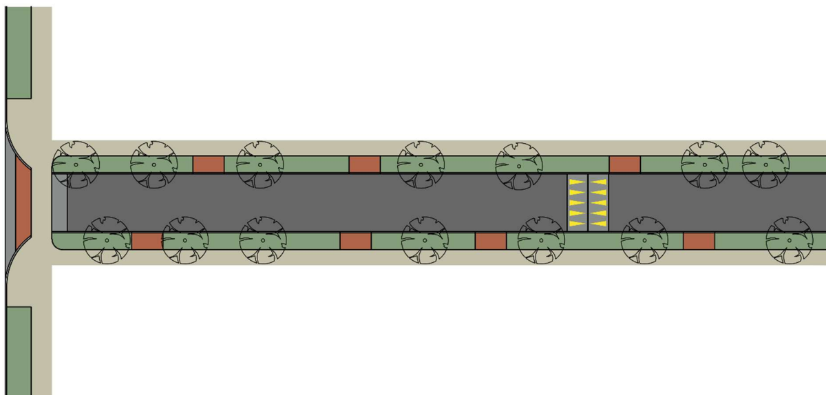
21. ábra: Minimális elemkészlettel jellemezhető lakóutca (példa)
