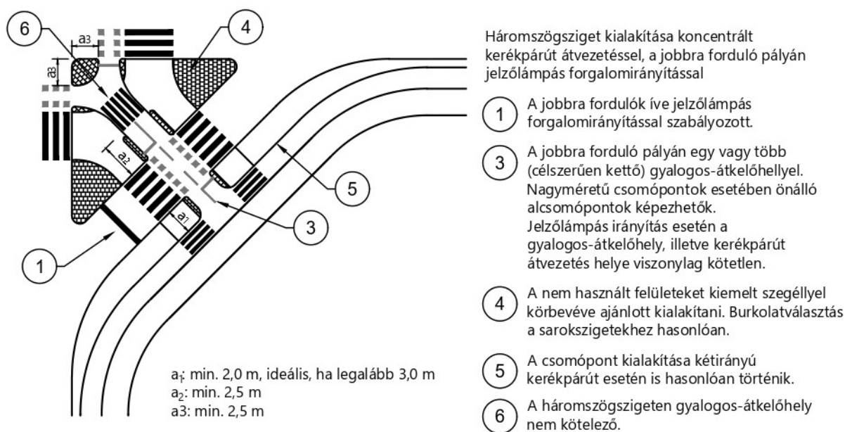
124. ábra: Háromszögsziget kialakítási lehetősége jelzőlámpás forgalomirányítás esetén (példa)
