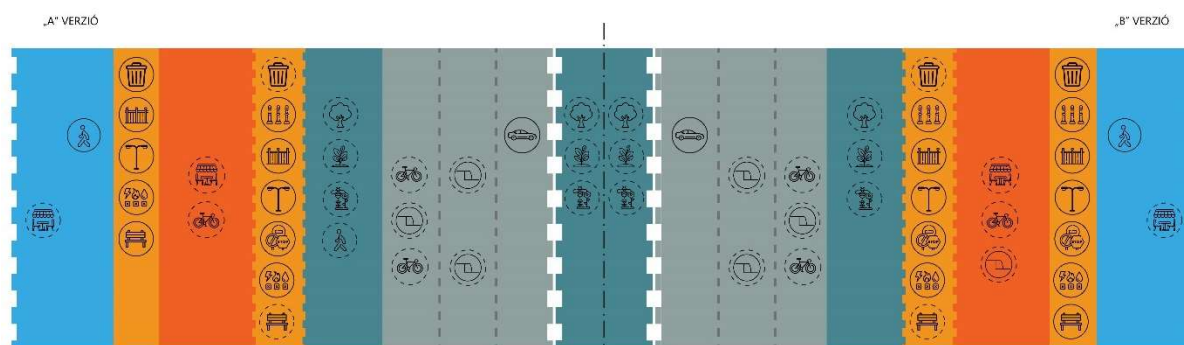
11. ábra: Emblematikus főút keresztmetszete
