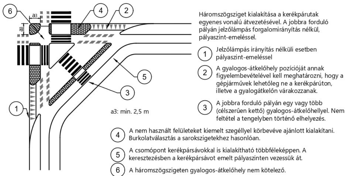
123. ábra: Háromszögsziget kialakítási lehetősége jelzőlámpa nélkül, elsősorban gyűjtőúti környezetben (példa)
