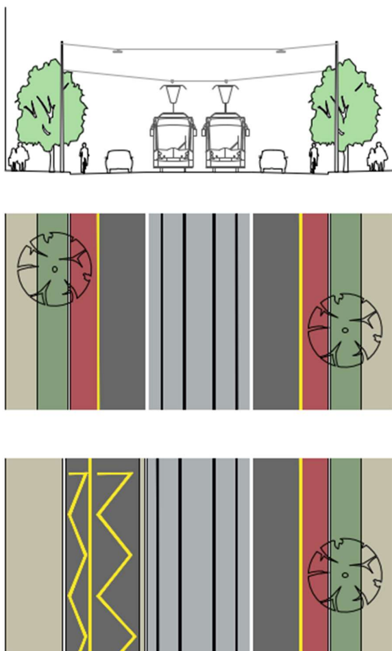
148. ábra: Úttestre történő leszállás elvi kialakítási lehetősége (példa)
