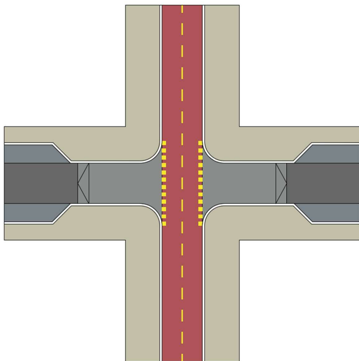
57. ábra: Elsőbbséggel átvezetett kerékpárút lakóúti környezetben (példa)
