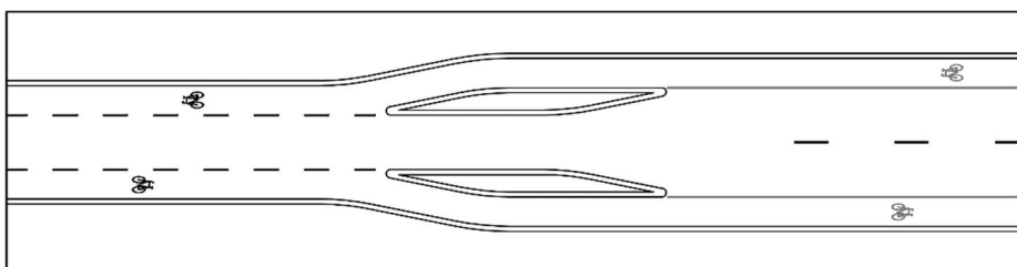
54. ábra: Nyitott kerékpársáv előtti átmenet útszűkítéssel (példa)
