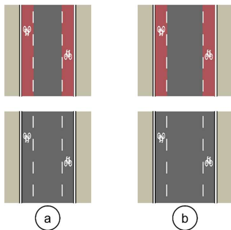
33. ábra: Nyitott kerékpársáv a kerékpársávok között legfeljebb 3,8 m széles felülettel (balra) és legalább 4,8 m széles felülettel (jobbra)
