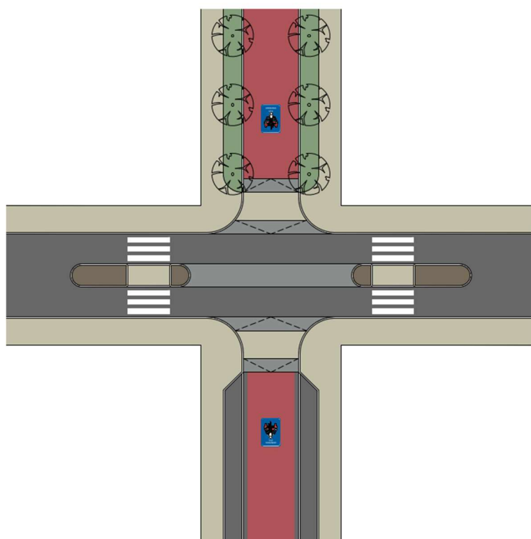
60. ábra: Kerékpáros utca és gyűjtőút keresztezésének kialakítása jelzőtáblával (példa)
