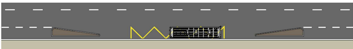
140. ábra: Öbolszerűen kialakított megállóhely a parkolósáv megszakításával (példa)
