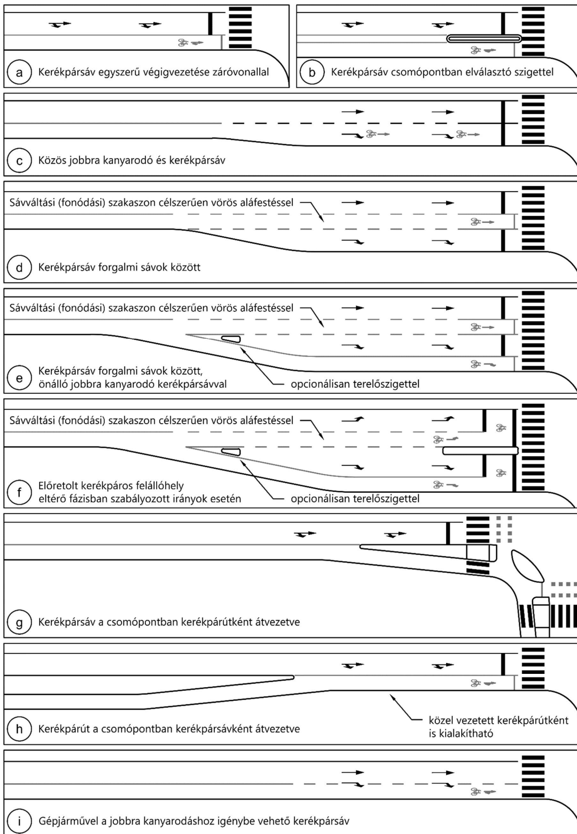
36. ábra: Irányhelyes kerékpárforgalmi létesítmények torkolati kialakításának változatai (példák)
