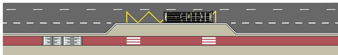
143. ábra: Félszigetes megállóhely kerékpárúttal (példa)
