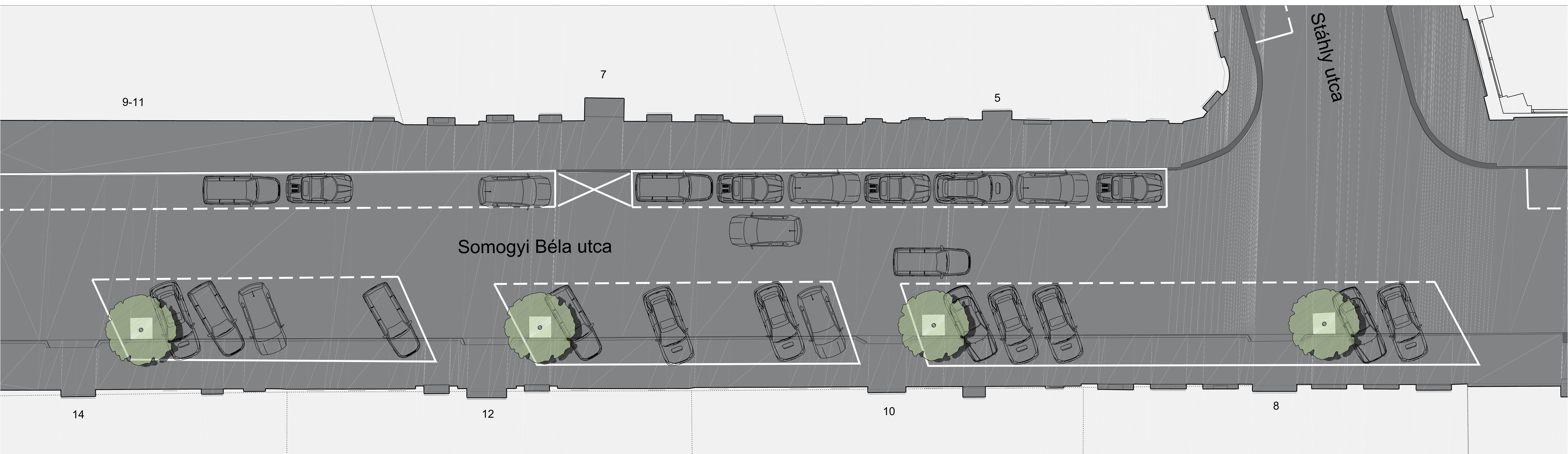
Tervezett állapot
